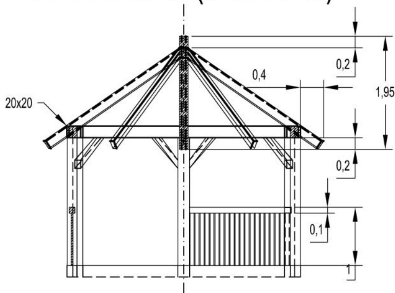
A-A metszet (szerkezet)
